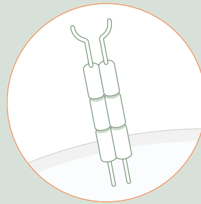
TCR GENERIERUNG
