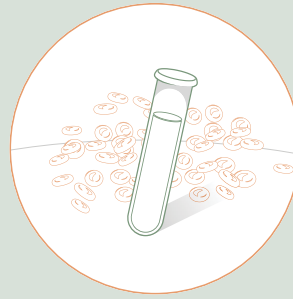
ZIELMOLEKÜL SCREENING
