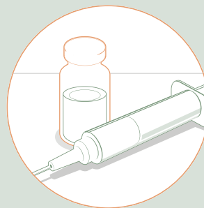
KLINISCHE ENTWICKLUNG
